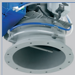
Вариант конструкции с обтекатель и фланцем
