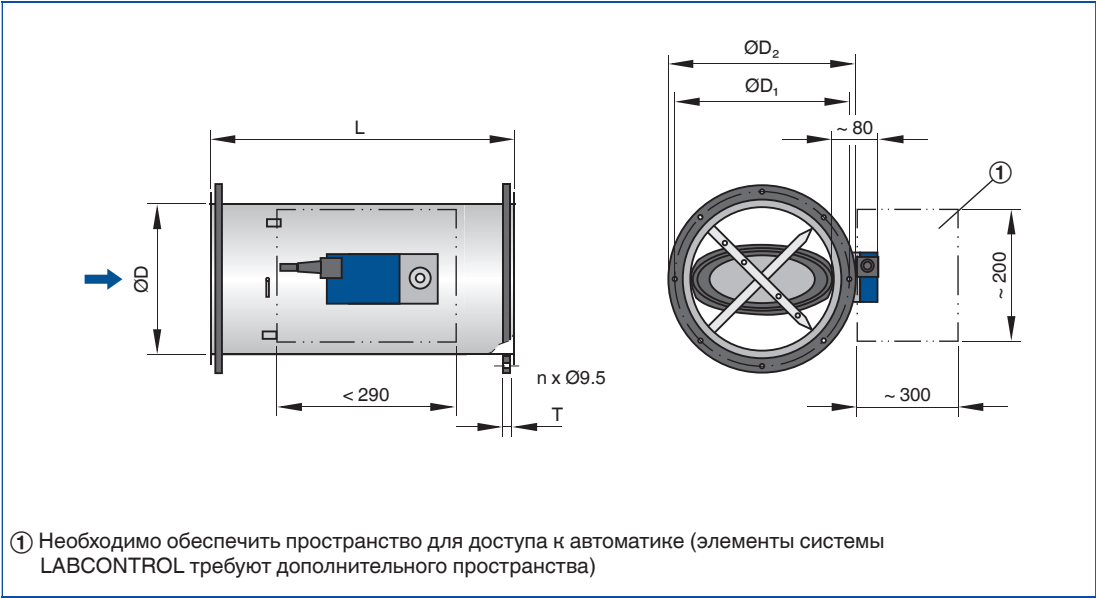
Чертеж PBAY-FL
